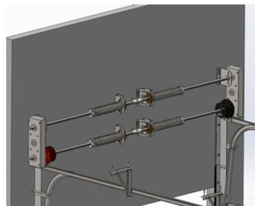
синхронизация с помощью редуктора
