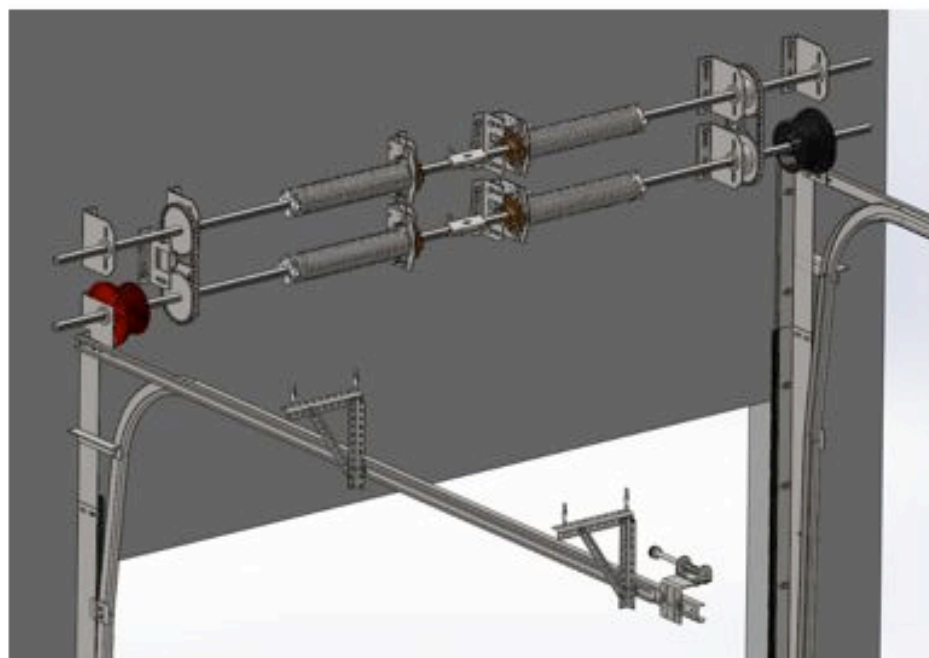
синхронизация с помощью цепи
